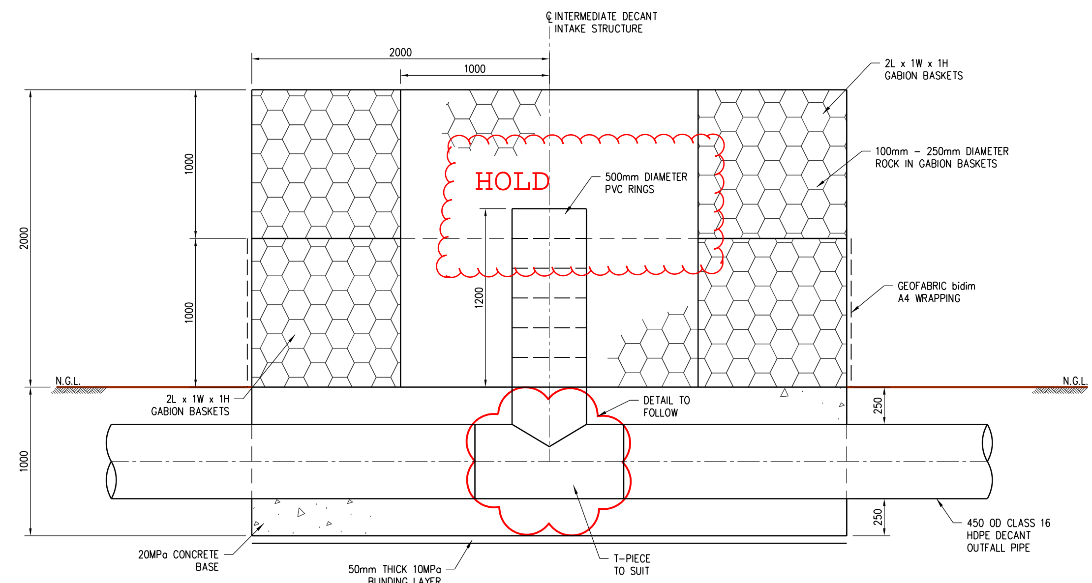
SECTION B 1:25
